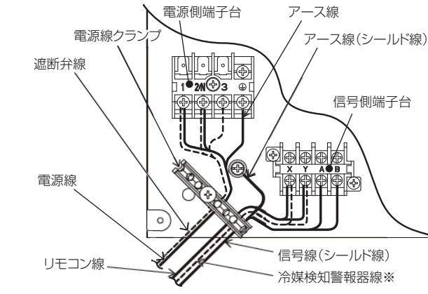
R32 ビル用マルチ機の配線接続
