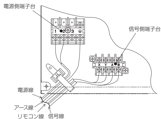
R410A ビル用マルチ機の配線接続
