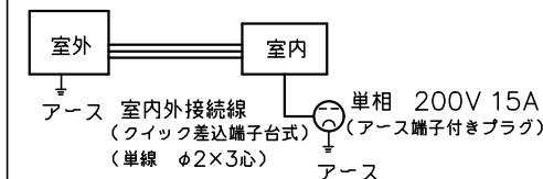
配線接続図
