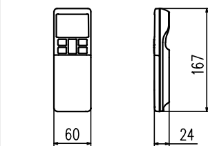
外形図（リモコン）
