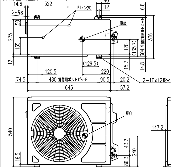
外形図（室外ユニット）
