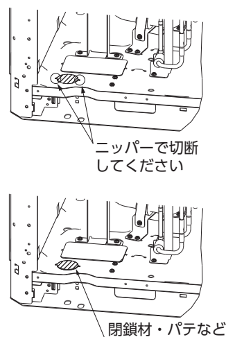
下面取出しの場合
