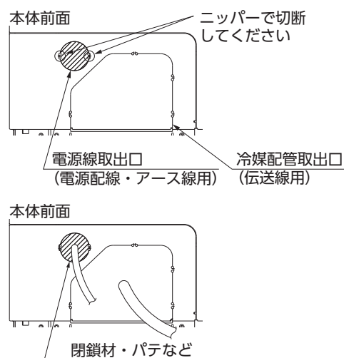
正面取出しの場合
