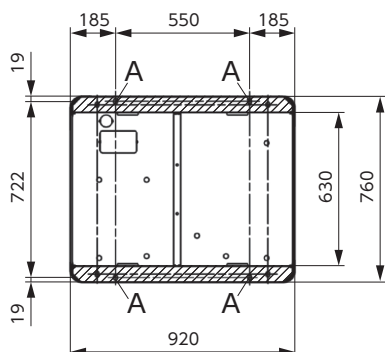
大母型(FDC(S)P500,5601LXZ/ FDC(S)P615, 6701LXZ-N)
