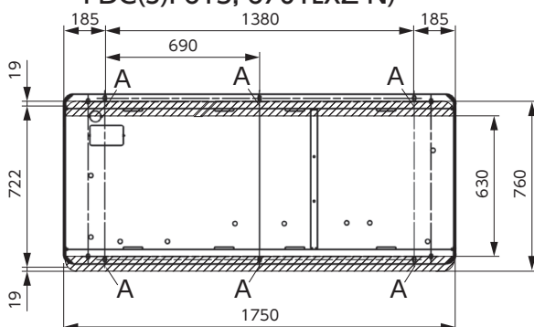
大母型(FDC(S)P500,5601LXZ/ FDC(S)P615, 6701LXZ-N)
