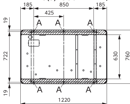
中母型(FDC(S)P335, 400, 4501LXZ/ FDC(S)P5001LXZ-N)
