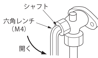
液管・均油管操作弁の開閉方法
