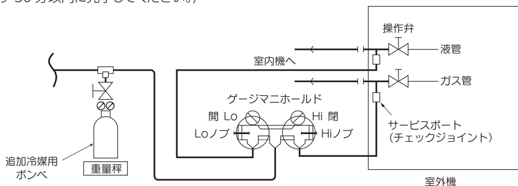
真空ポンプ接続例
