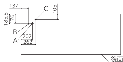
冷媒配管接続口の寸法(平面図)
