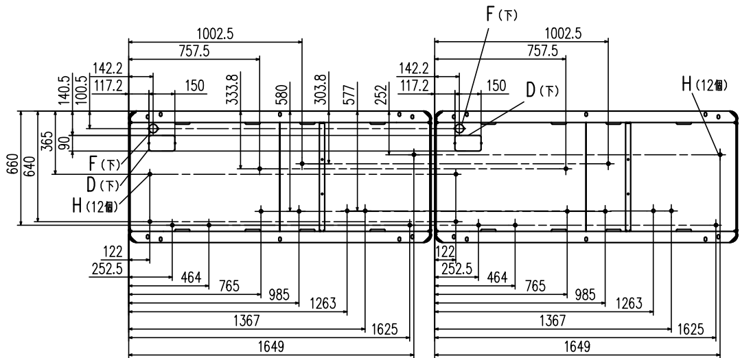
冷媒配管取出口、電源取入口、ドレン排水用穴寸法
