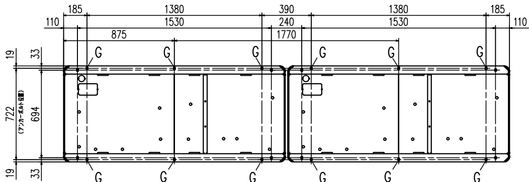
アンカーボルト用穴寸法
