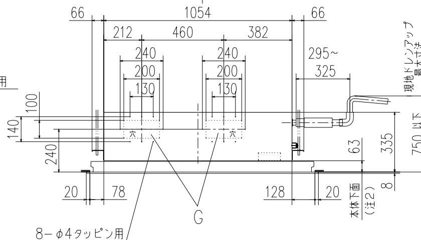
据付スペース
