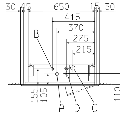
据付スペース
