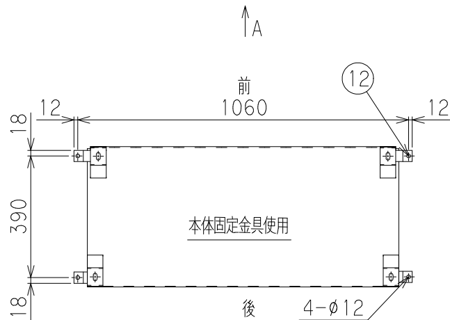
A矢視 (本体固定方法詳細)
