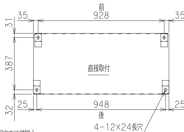
A矢視 (本体固定方法詳細)
