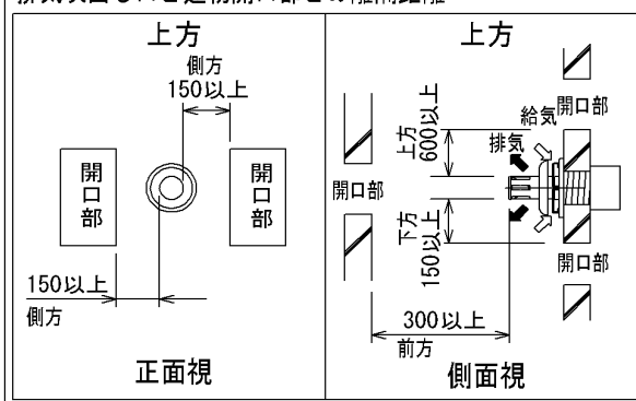
排気吹出し口と建物開口部との離隔距離
