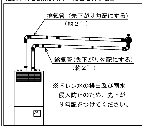
延長部材を複数使用して配管を行う場合
