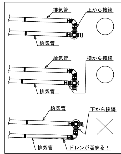
延長部材を複数使用して配管を行う場合の注意事項
