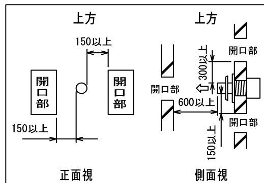
排気吹出し口と建物開口部との離隔距離 単位:mm
