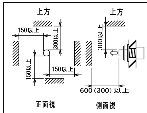
排気吹出し口と周囲構造物との離隔距離 ※(300)は不燃材料で有効に仕上げた場合
