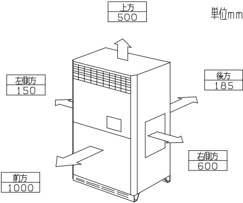
暖房機と周囲構造物との離隔距離
