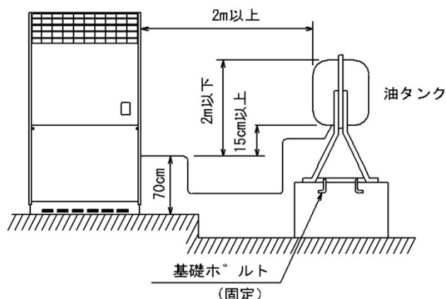
【200ℓ未満の油タンクの場合】
