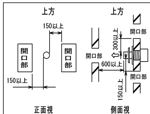
排気吹出し口と建物開口部との離隔距離 単位: mm
