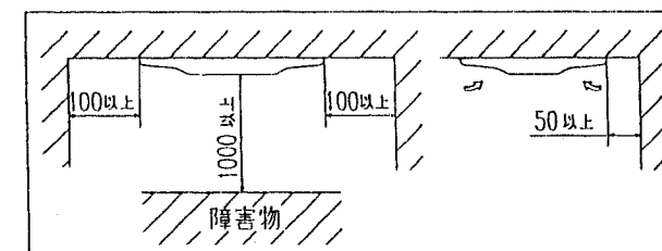
据付スペース
