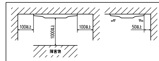
据付スペース
