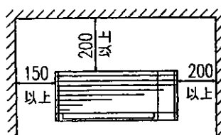
据付スペース
