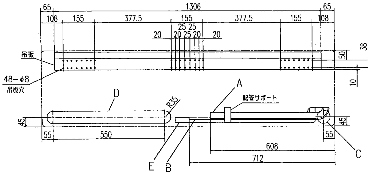
正面から見た据付け位置図
