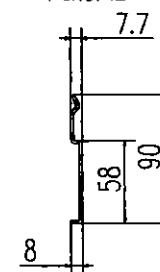
吊板詳細
