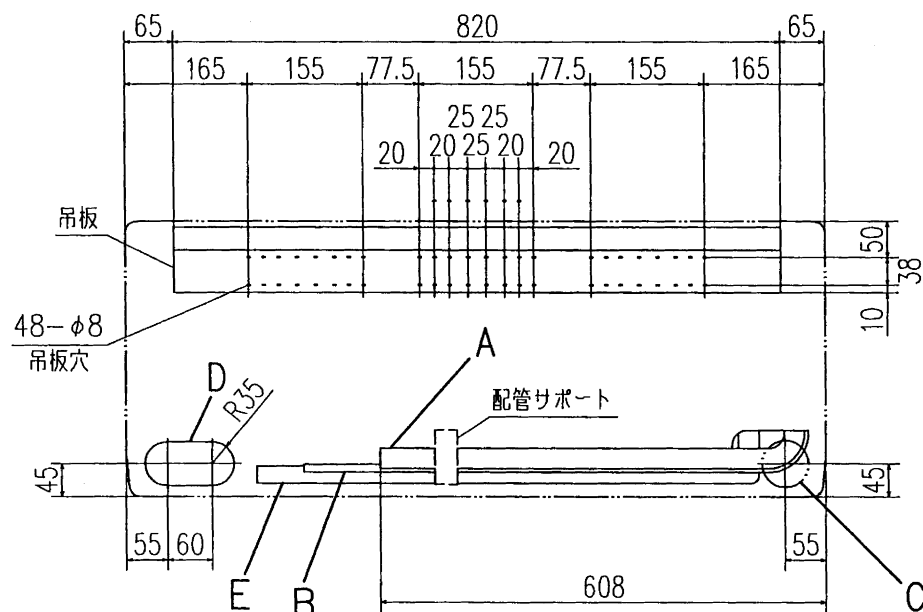
正面から見た据付け位置図
