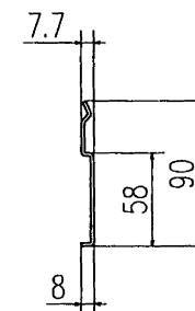
吊板詳細
