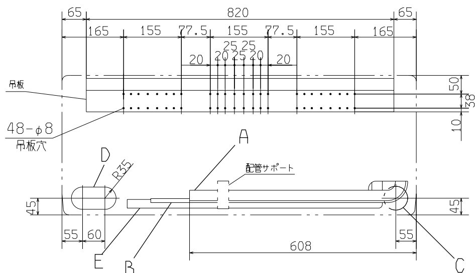
正面から見た据付け位置図
