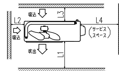
据付最小スペース
