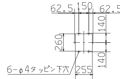
Z (側面詳細)
