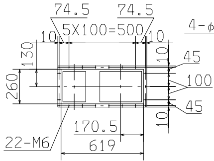
X (送風機室天井詳細)
