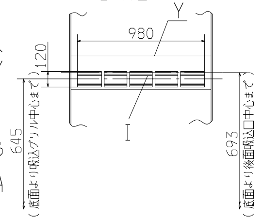
Z (後面)
