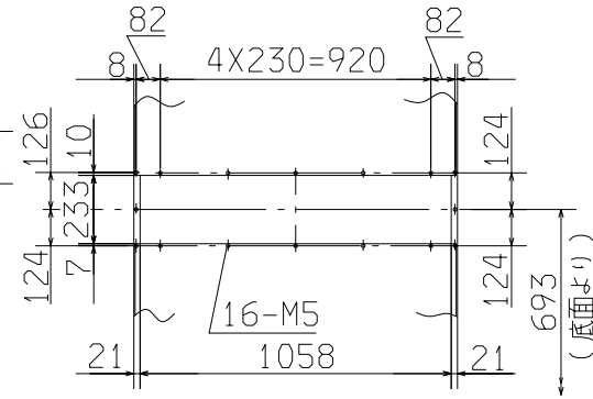
Y (後面吸込口詳細)
