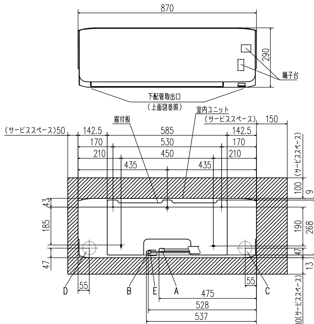
正面から見た据付け位置図及び据付けスペース
