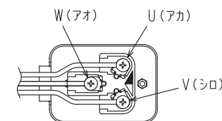
※圧縮機端子拡大図
