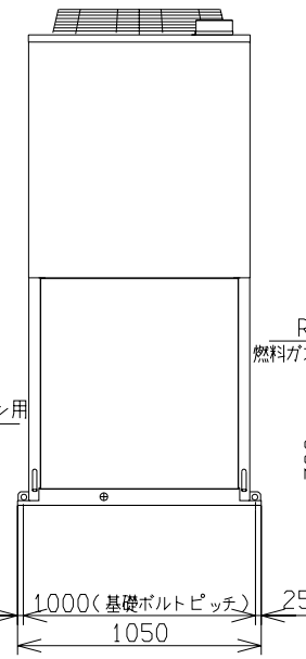
右側面図
