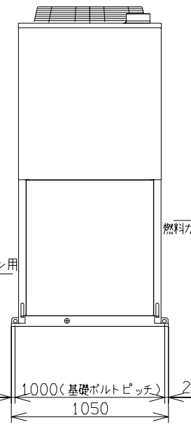
右側面図
