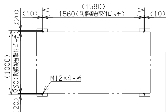
防振架台の取付寸法
