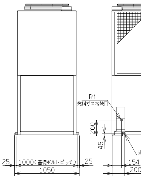
右側面図
