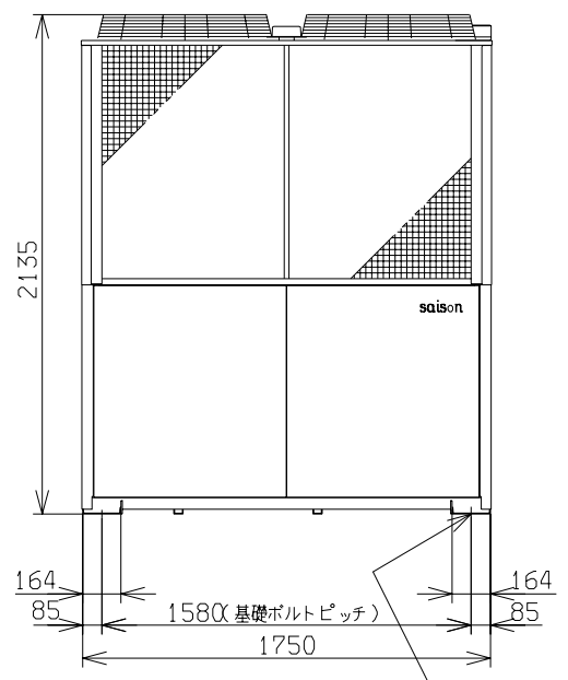
正面図
