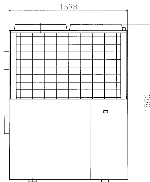
正面図
