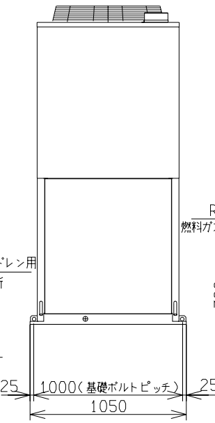
右側面図
