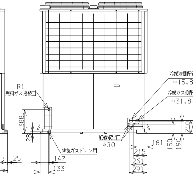
背面図
