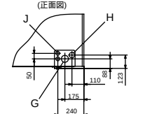
冷媒配管接続口の寸法 (正面図)
