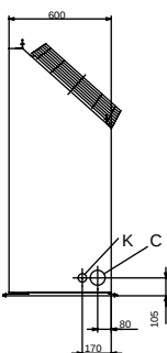
冷媒配管接続口の寸法 (正面図)
