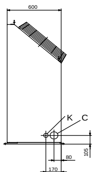
冷媒配管接続口の寸法 (正面図)
