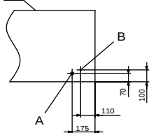
冷媒配管接続口の寸法 (後面 (平面図))
