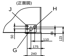
冷媒配管接続口の寸法 (正面図)
