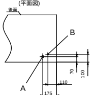
冷媒配管接続口の寸法 (後面 (平面図))
