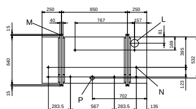
冷媒配管接続口の寸法 (正面図)
