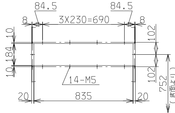
Y (後面吸込口詳細)
