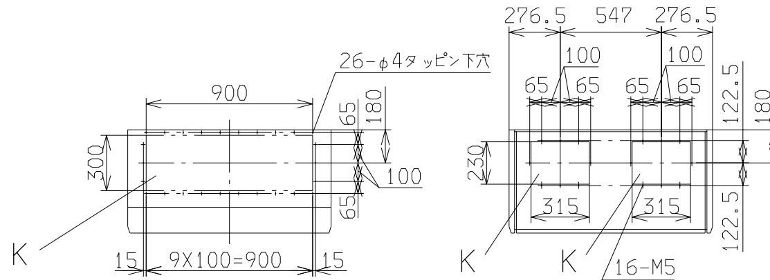
Z-Z (送風機室天井詳細)
