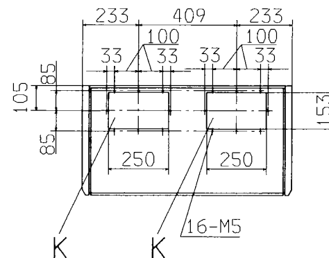
Z-Z (送風機室天井詳細)
