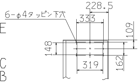
Y (側面詳細)
