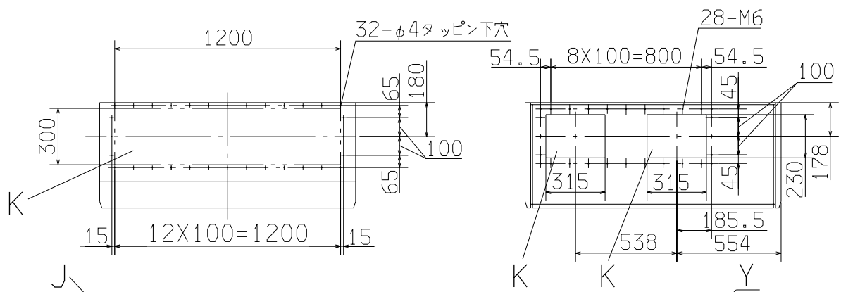
Z-Z (送風機室天井詳細)
