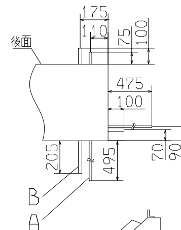
付属冷媒配管接続後の寸法(平面図)
