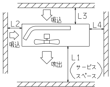
据付スペース (単位: mm)
