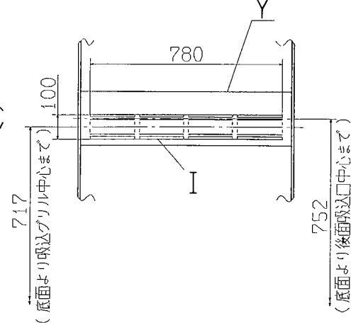
Z (後面)
