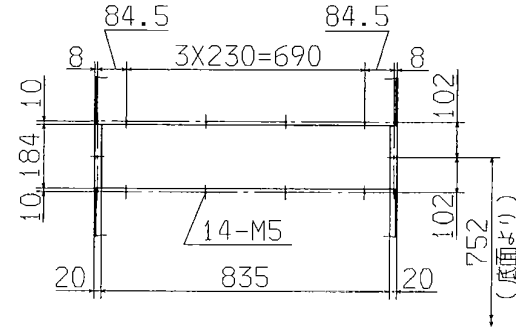
Y (後面吸込口詳細)
