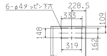
W (側面詳細)
