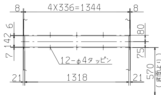
Y (後面吸込口詳細)
