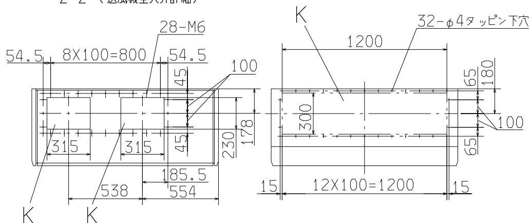
Z-Z (送風機室天井詳細)
