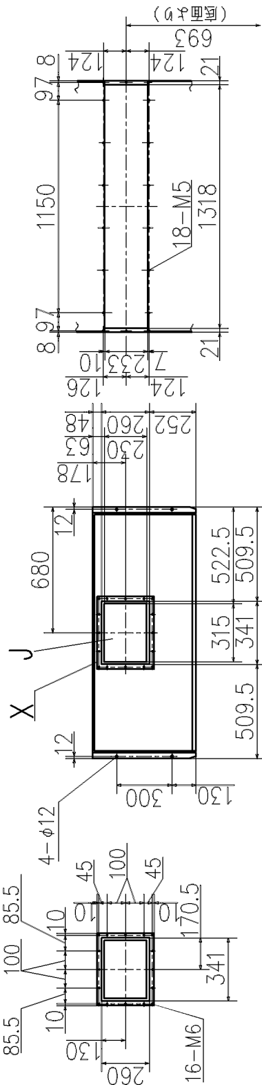
Y (後面吸込口詳細)
