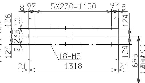
Y (後面吸込口詳細)
