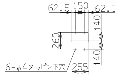
Z (側面詳細)
