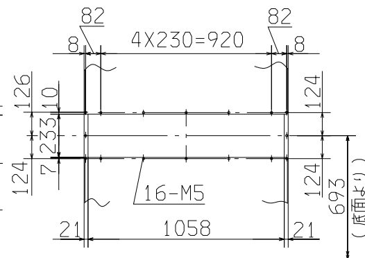
Y (後面吸込口詳細)
