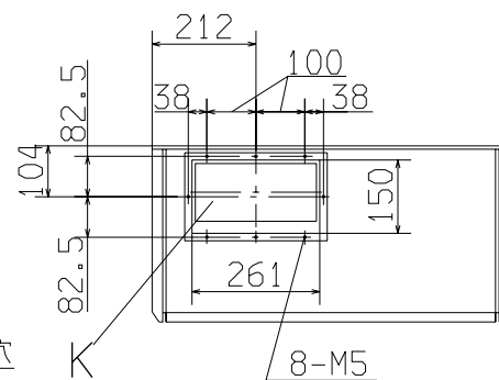
Z-Z (送風機室天井詳細)
