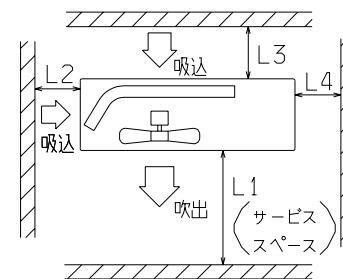
据付スペース (単位: mm)
