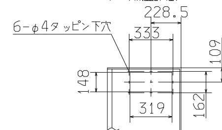
Y (側面詳細)
