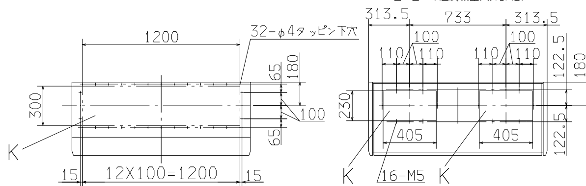
Z-Z (送風機室天井詳細)
