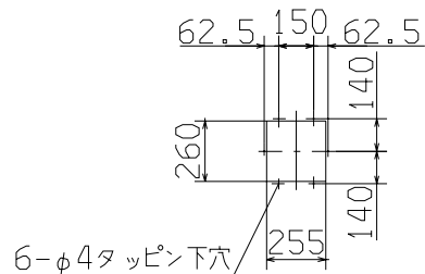
Z (側面詳細)
