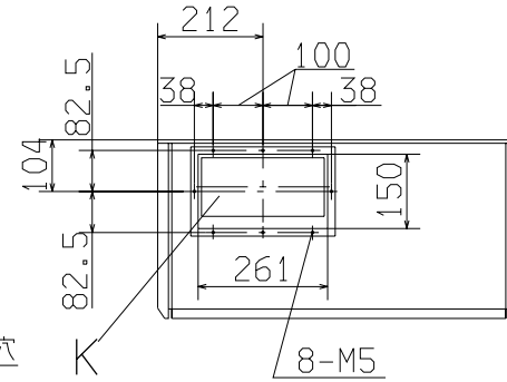
Z-Z (送風機室天井詳細)
