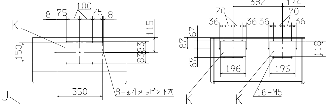
Z-Z (送風機室天井詳細)
