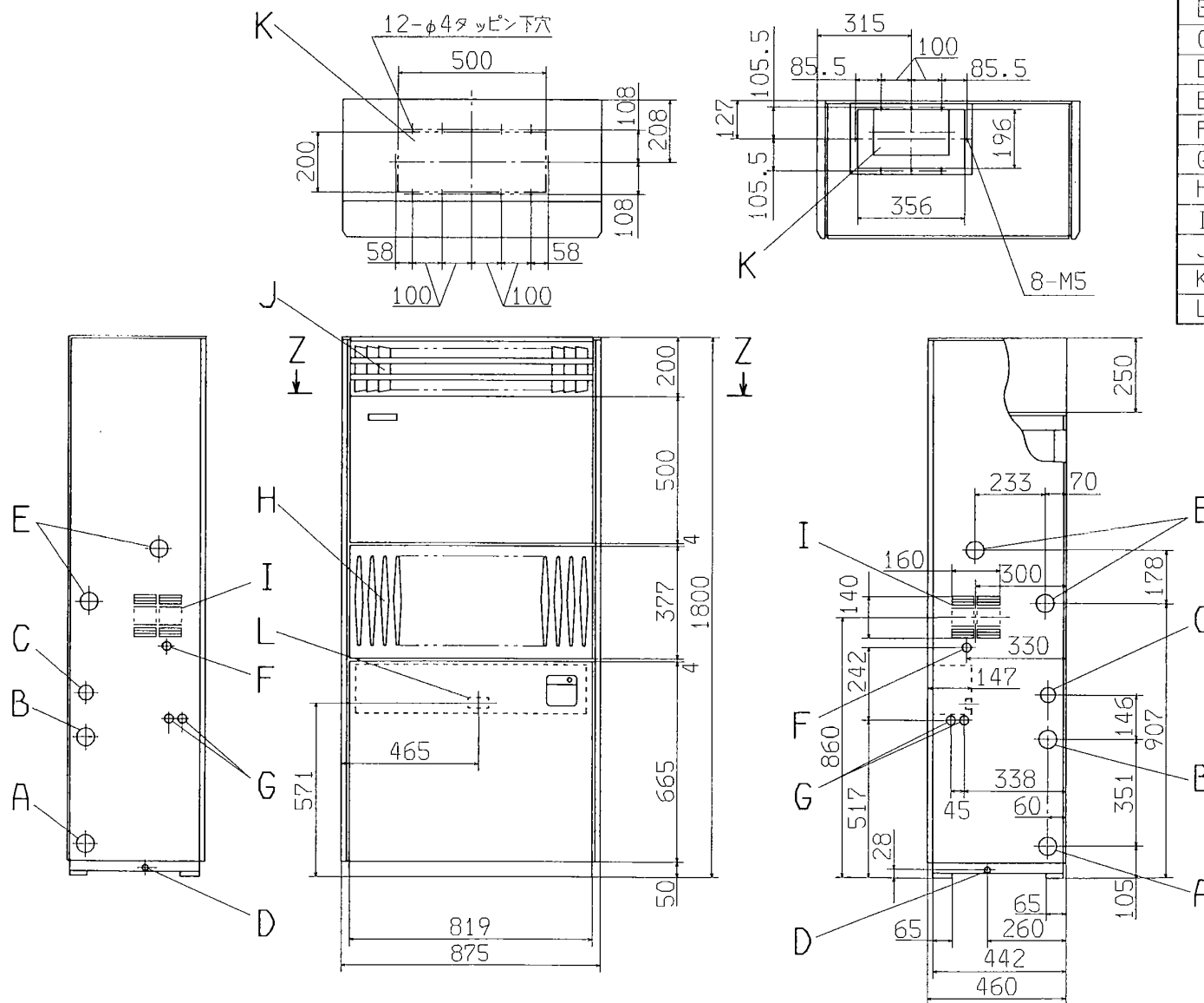
Z-Z (送風機空天井詳細)
