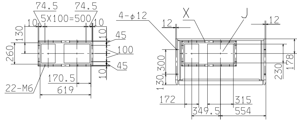
X (送風機室天井詳細)
