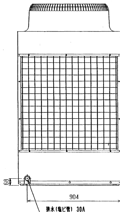
背面図
