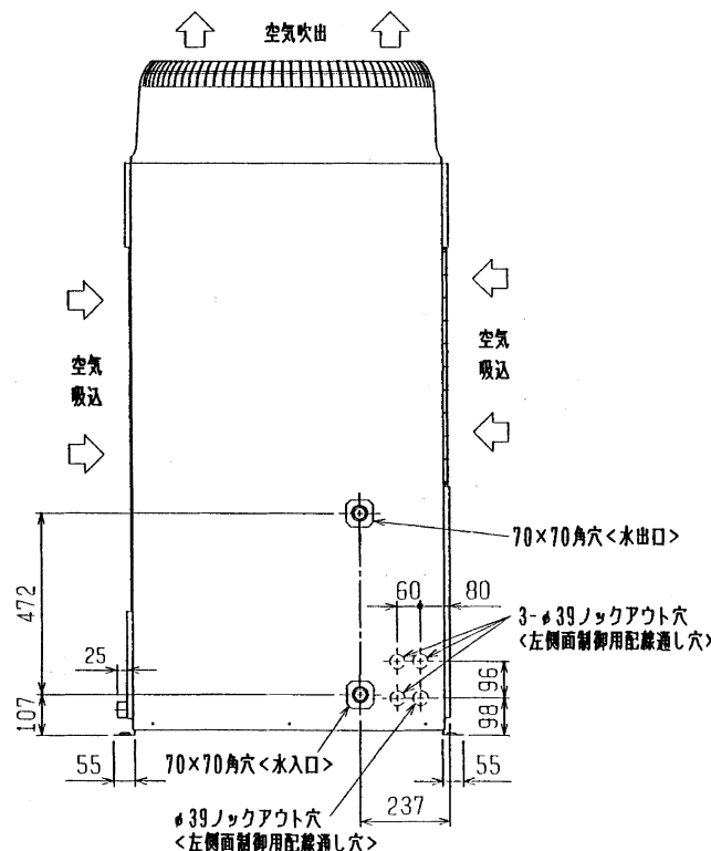
左側面図
