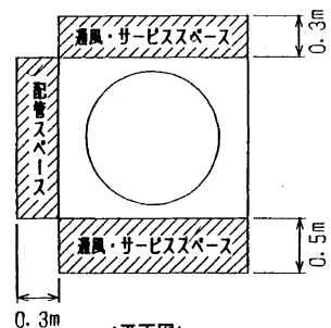
＜平面図＞ サービススペース
