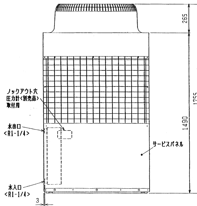
正面図
